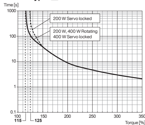
• Motor Type : □ 60 mm MHMG
