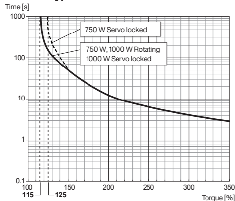
• Motor Type : □ 80 mm MHMG
