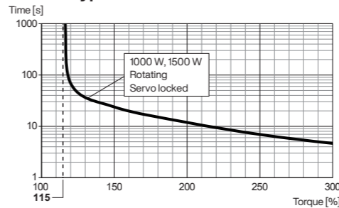
• Motor Type : □ 130 mm MDMG
