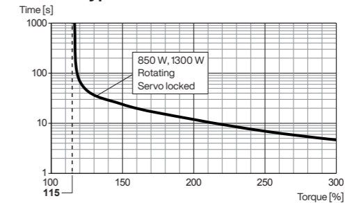
• Motor Type : □ 130 mm MGMG
